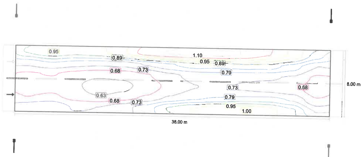
Observator 1: Valoarea de întreținere, densitatea luminii cu carosabil uscat [ cd/m^2 ] (Linii Isolux)
