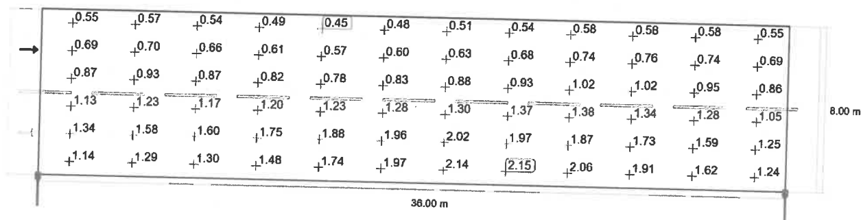
Observator 2: Valoarea de întreținere, densitatea luminii cu carosabil uscat [ \text{cd}/\text{m}^2 ] (Raster valoric)
