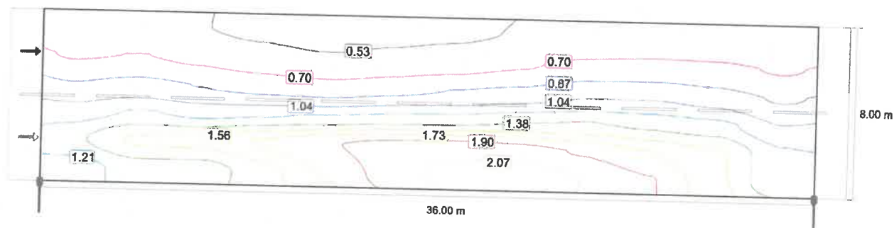
Observator 2: Valoarea de întreținere, densitatea luminii cu carosabil uscat [ \text{cd}/\text{m}^2 ] (Linii Isolux)
