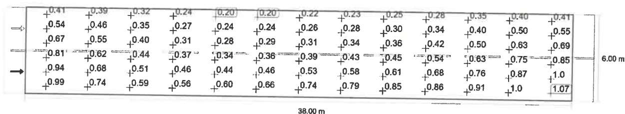
Observator 1: Valoarea de întreținere, densitatea luminii cu carosabil uscat [ \text{cd}/\text{m}^2 ] (Linii Isolux)
